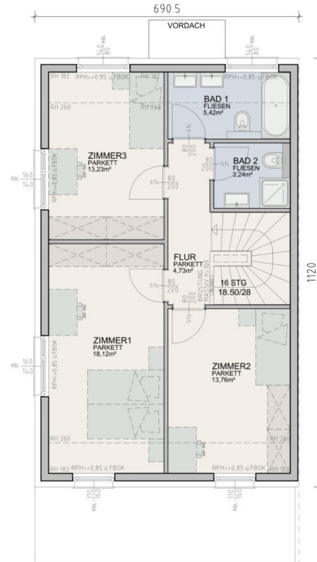
OBERGESCHOSS
